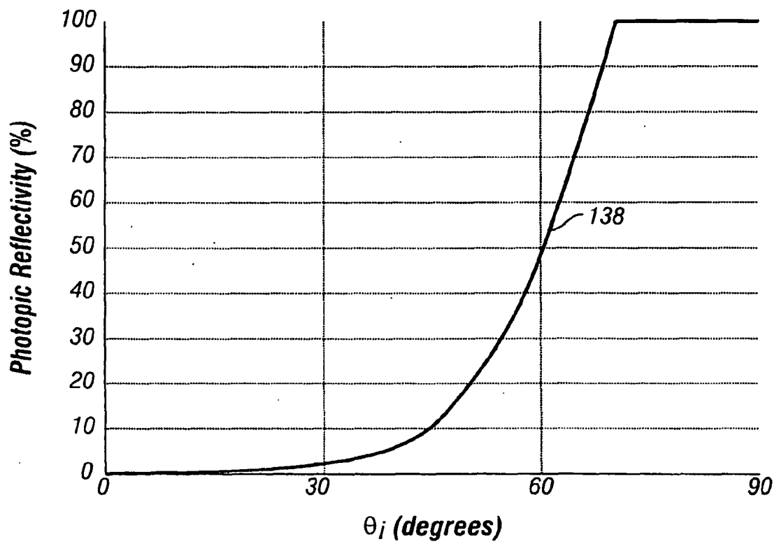
FIG. 13C
