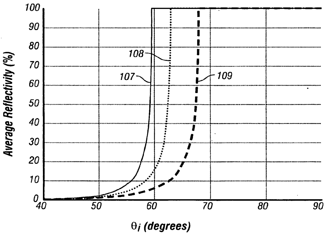
FIG. 10C
