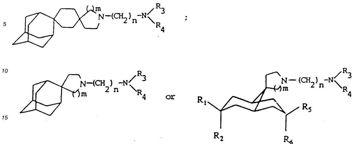
Formules (II)
