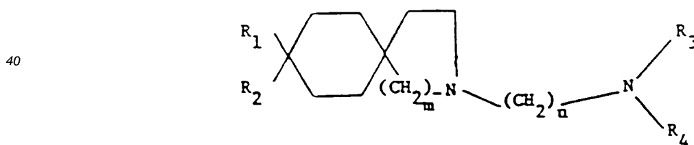
Formule (I)
