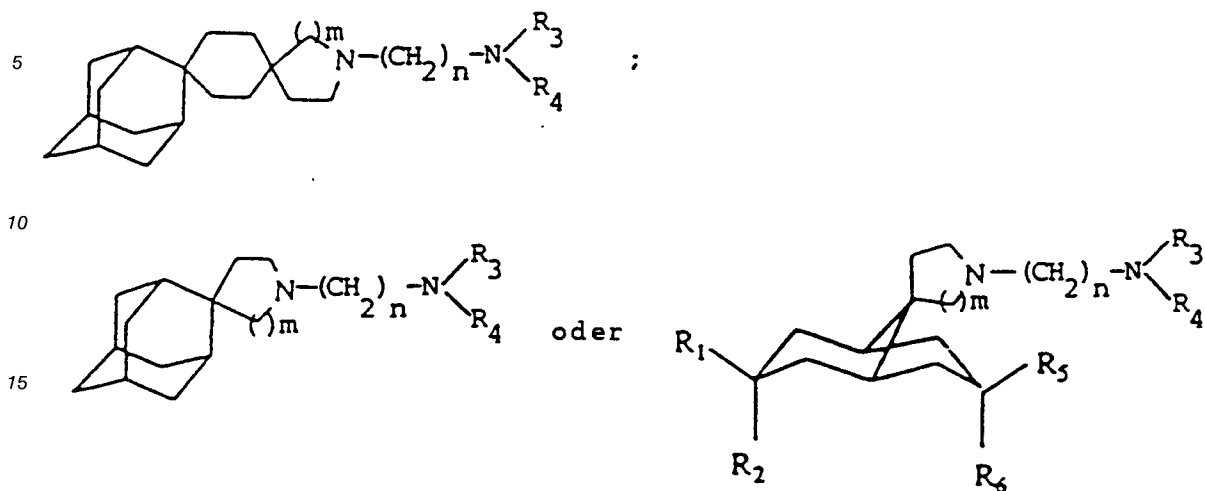
Formeln (II)
