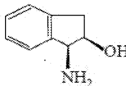
(-)-cis-1-amino-2-indanol (AI)
