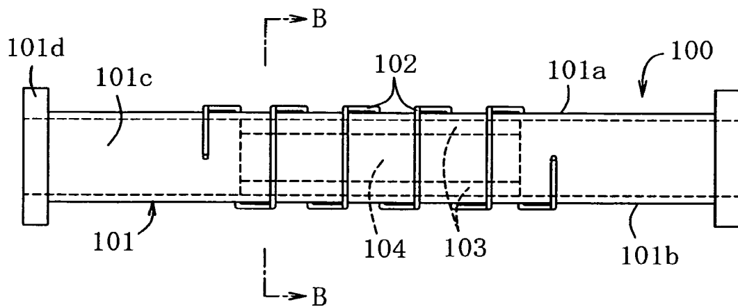
Fig. 19 -- Prior Art --
