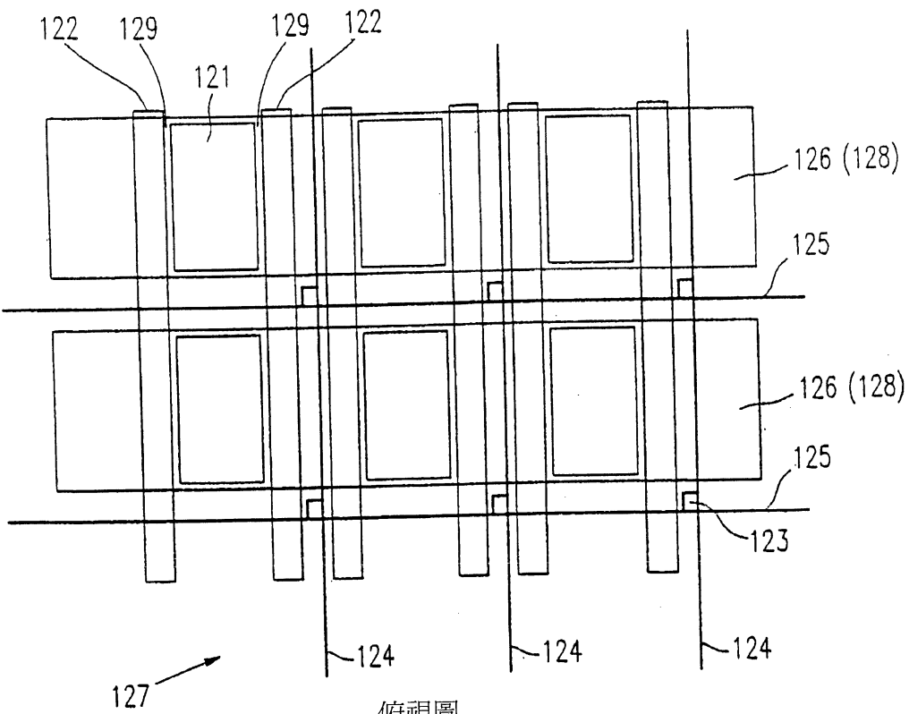
俯視圖 第 12A 圖
