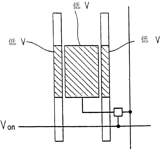
彩色狀態 第 12C-1 圖
