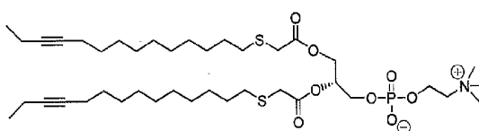
tTTA-PC 20
