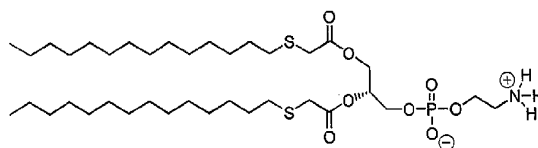
TTA-PE 21
