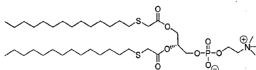
TTA-PC 18
