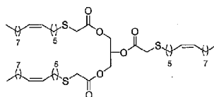
TTA-TAG 25
