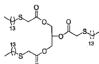
TTA-TAG 24
