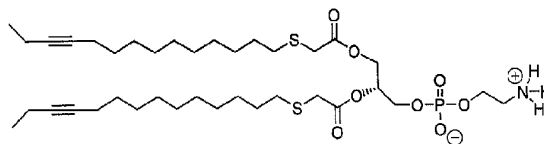
tTTA-PE 23
