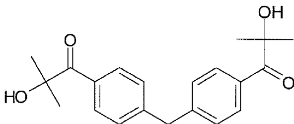
2-ヒドロキシ-1-[4-[4-(2-ヒドロキシ-2-メチル-プロピオニル)-ベンジル]フェニル]-2-メチル-プロパン-1-オン
