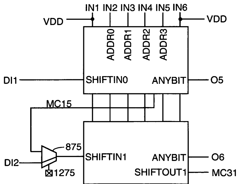
FIG. 13 (16x2 SRL)
