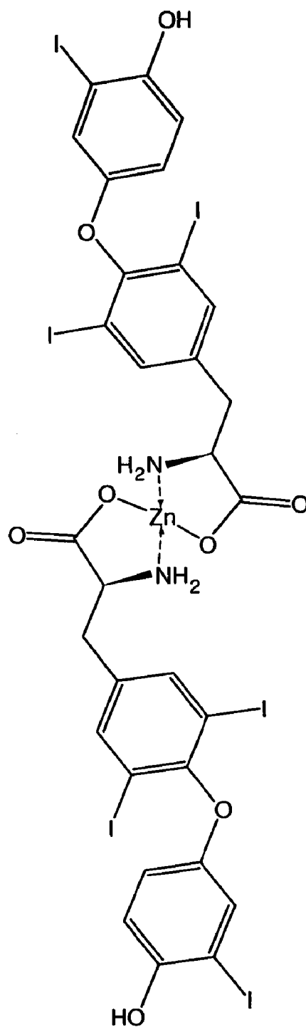
Bis(triiodothyroninato)zinc
