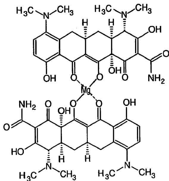
Bis(minocyclinato)magnesium
