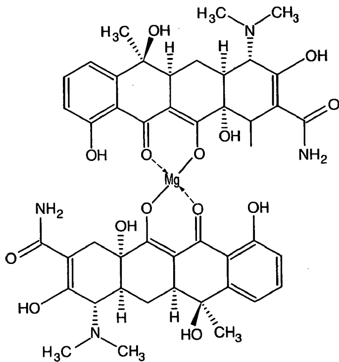
Bis(tetracyclinato)magnesium
