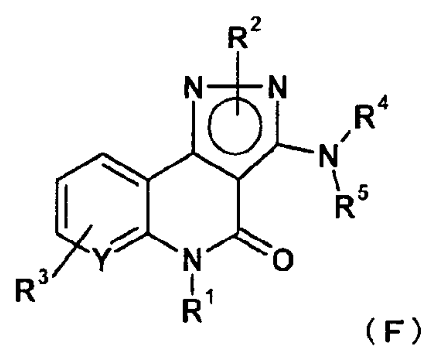
[Chem. 6]
