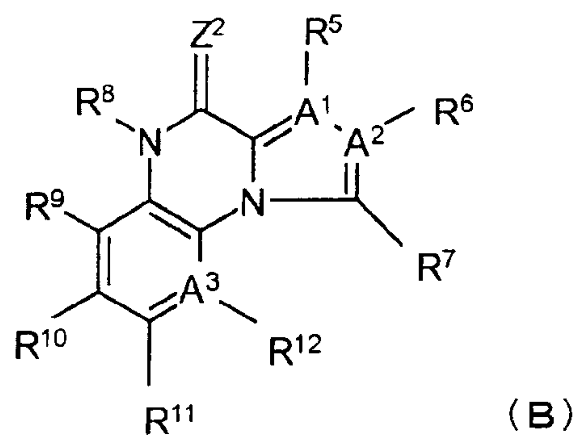
[Chem. 3]
