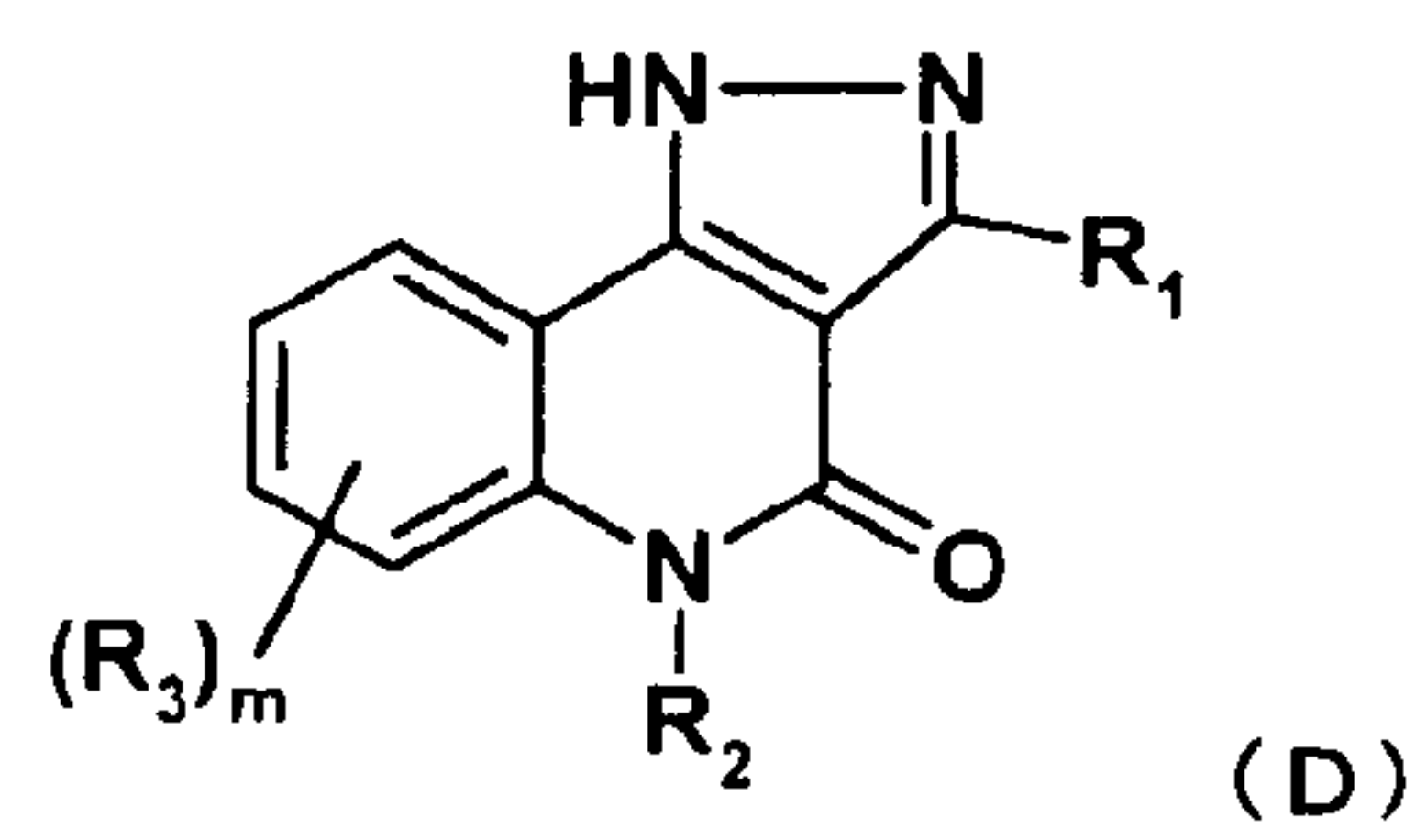
[Chem. 5]
