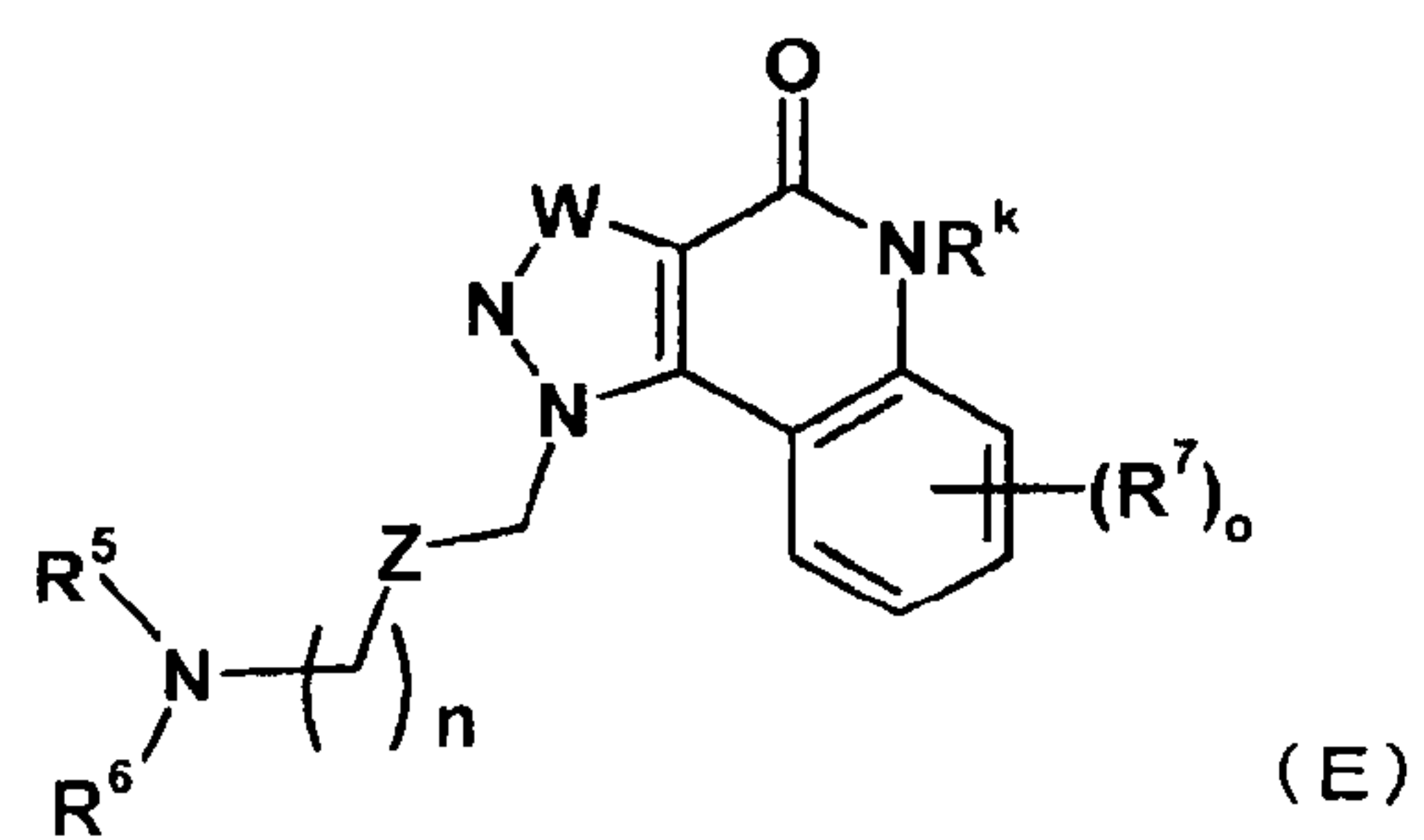
[Chem. 5]
