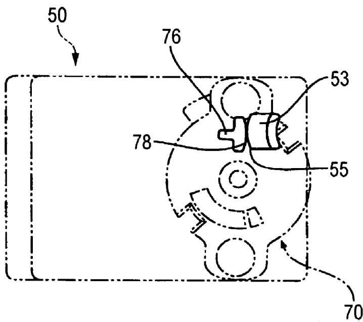
FIG. 11B
