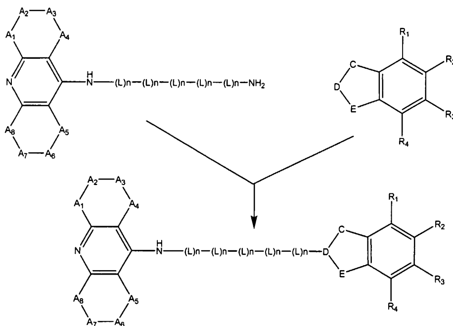
SCHEME 1a
