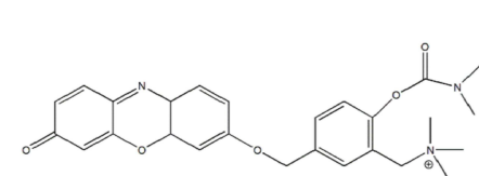
[화학식 12]
