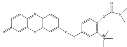
[화학식 11]
