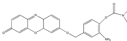
[화학식 12]
