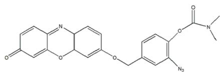
[화학식 11]
