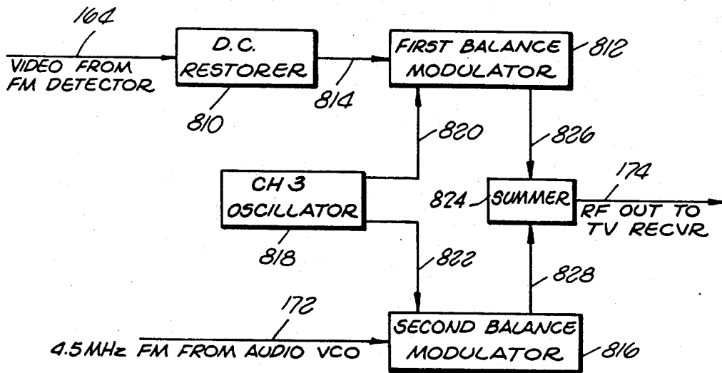
FIG. 24 RF MODULATOR
