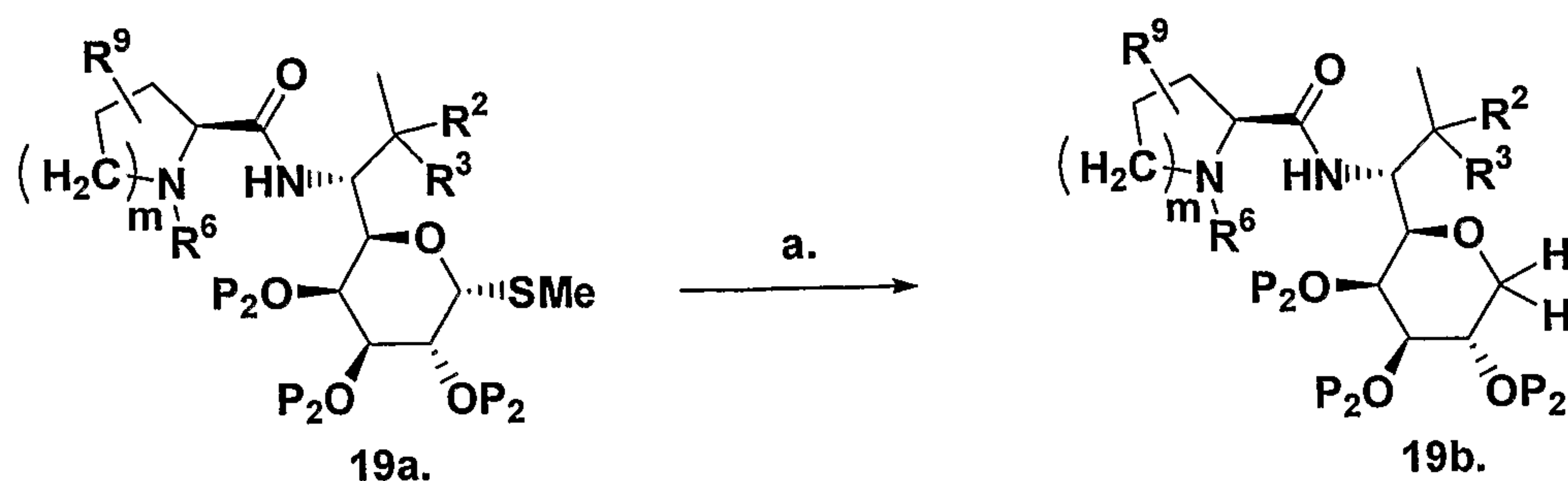
Scheme 20. a. Raney Nickel 2400, EtOH, reflux.
