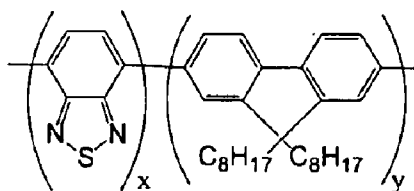
Poly(2,7-(9,9-di-n-octylfluorene)-benzothiadiazole)
