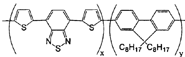
Poly(2,7-(9,9-di-n-octylfluorene)-(4,7-di-2-thienyl-(benzothiadiazole)))
