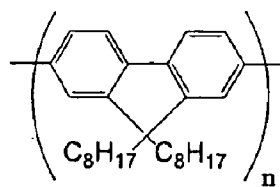
Poly(2,7-(9,9-di-n-octylfluorene)
