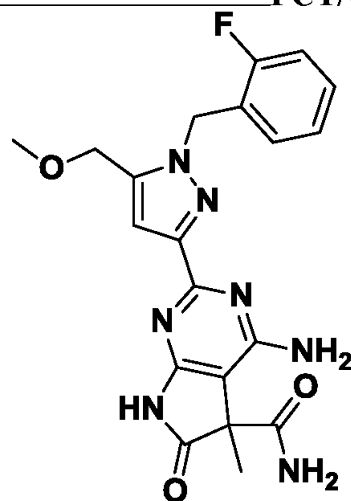
I-22
