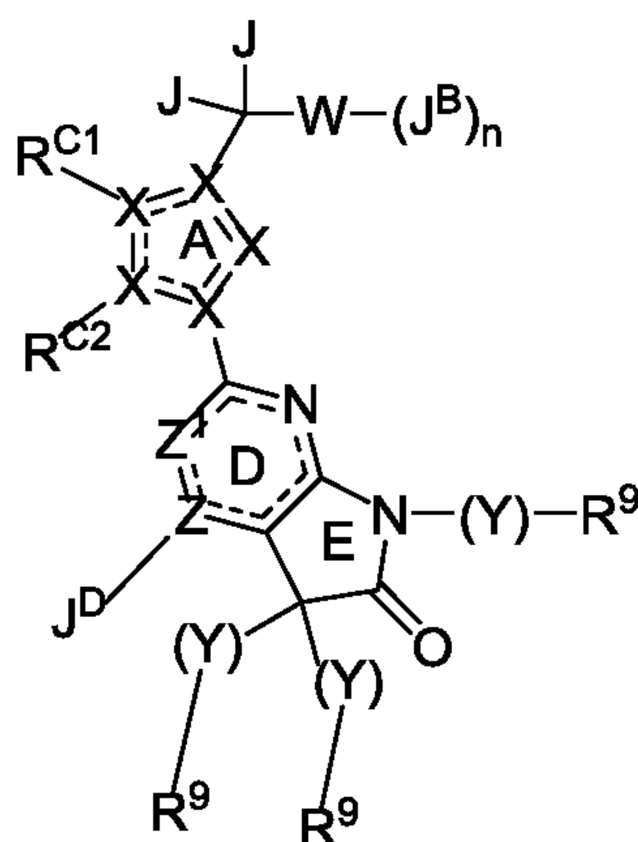
Formula I'B .
