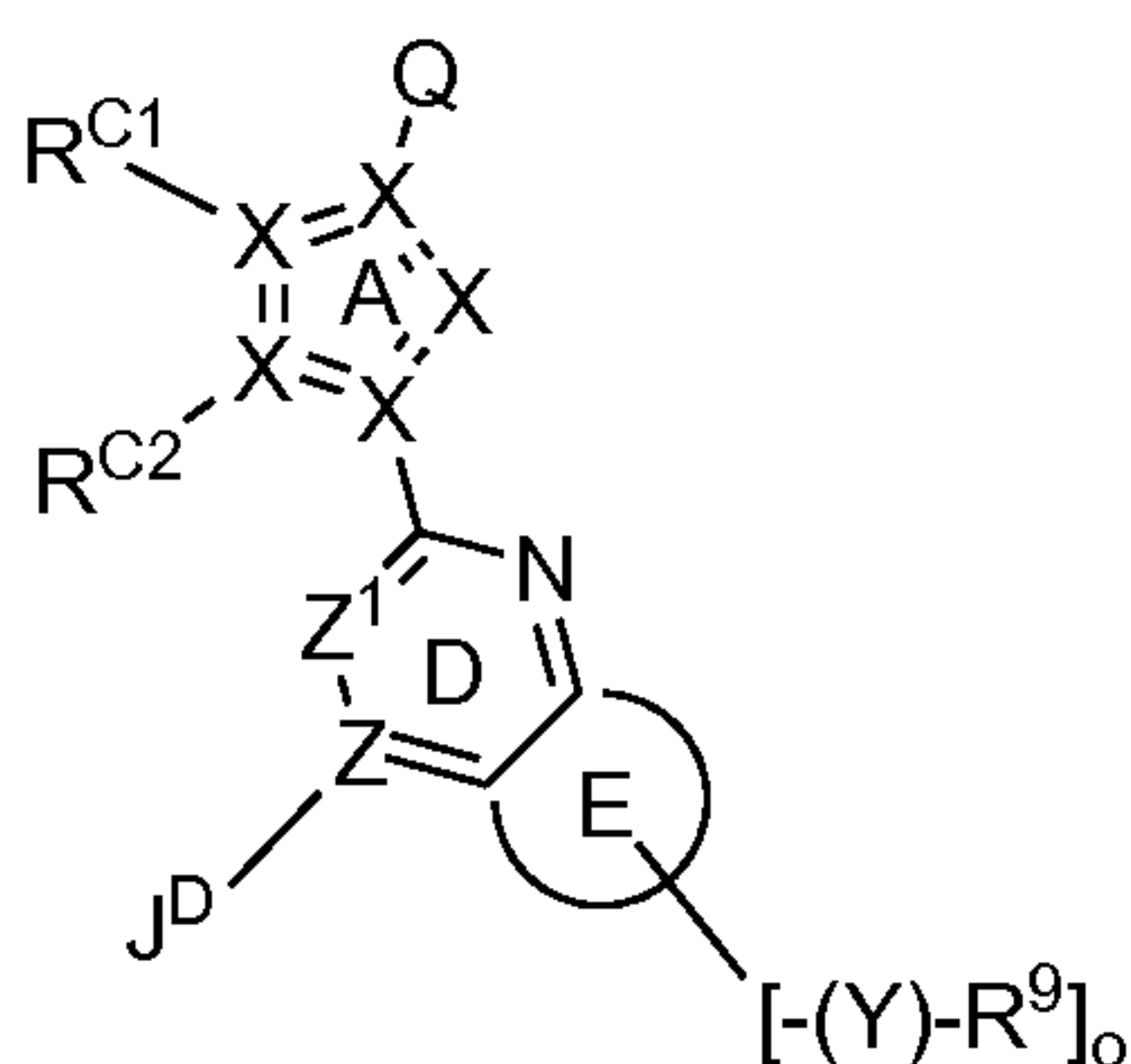
Formula I-a
