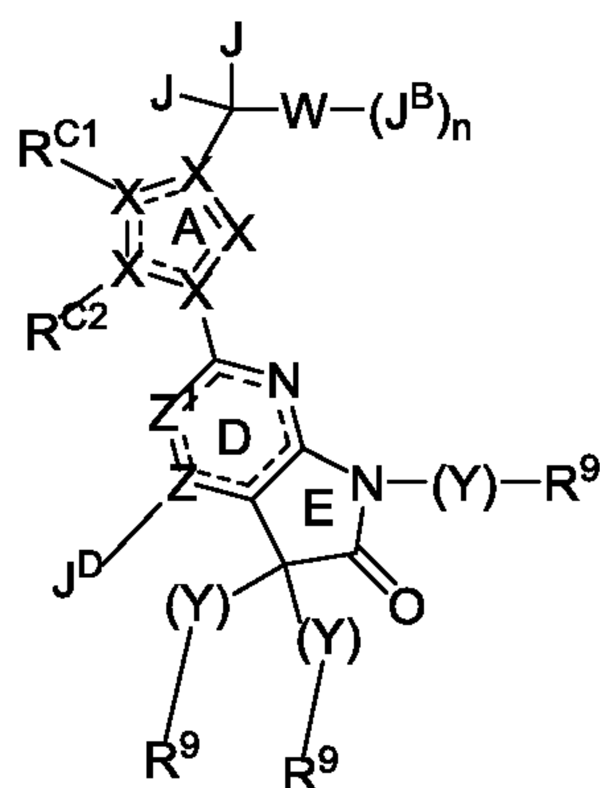
Formula I'B
