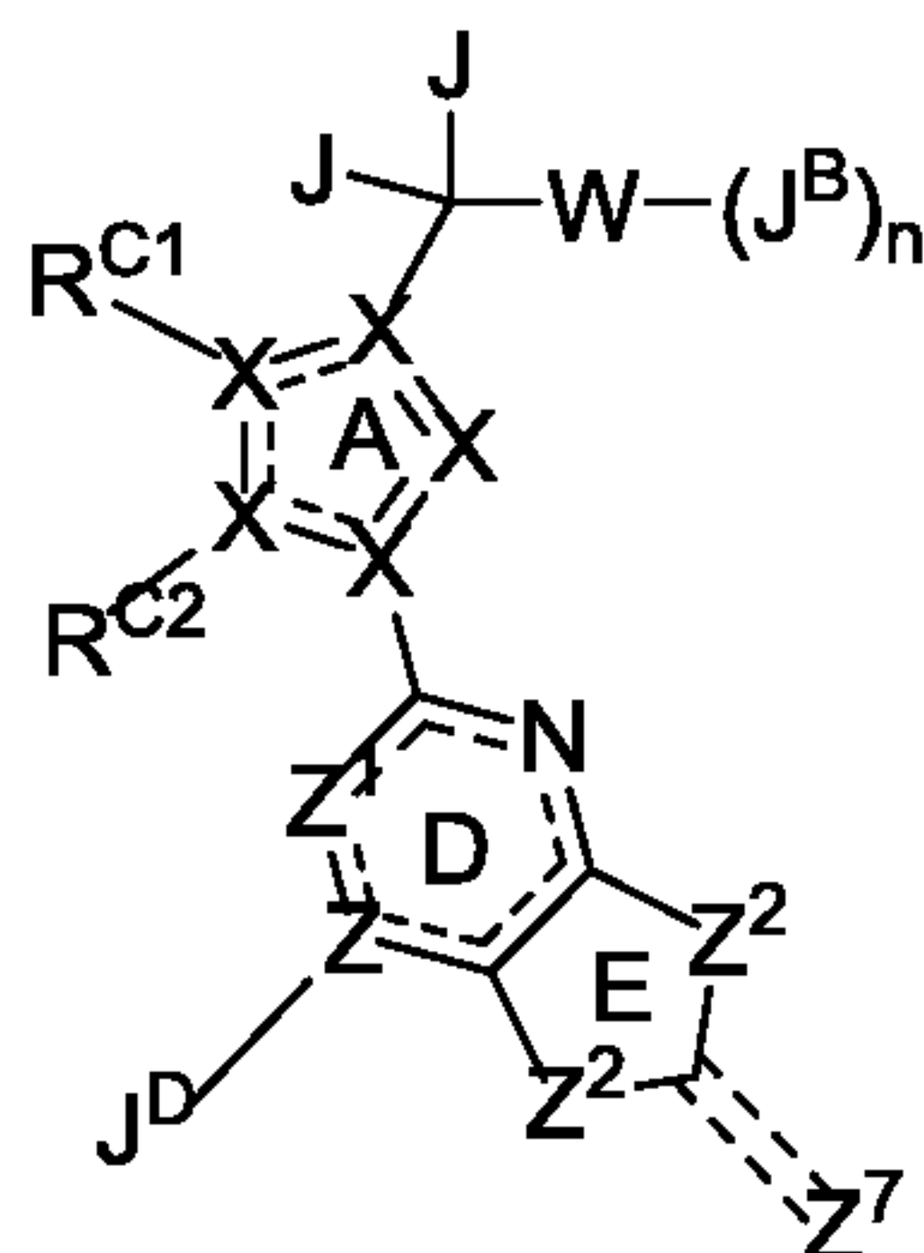
Formula I'A .
