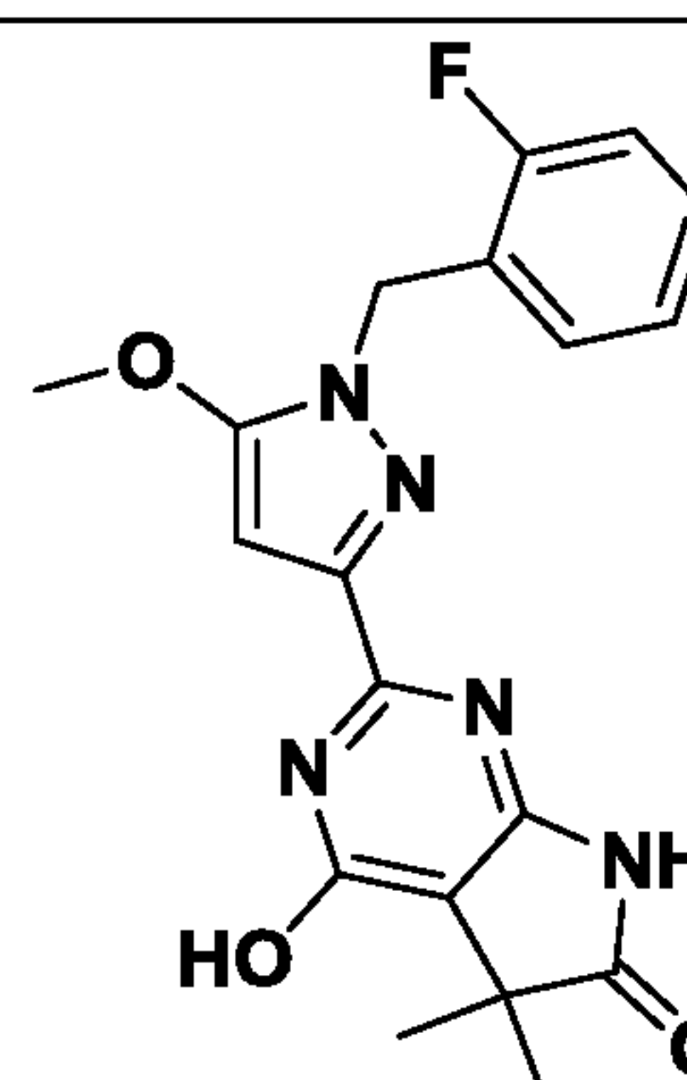
I-28
