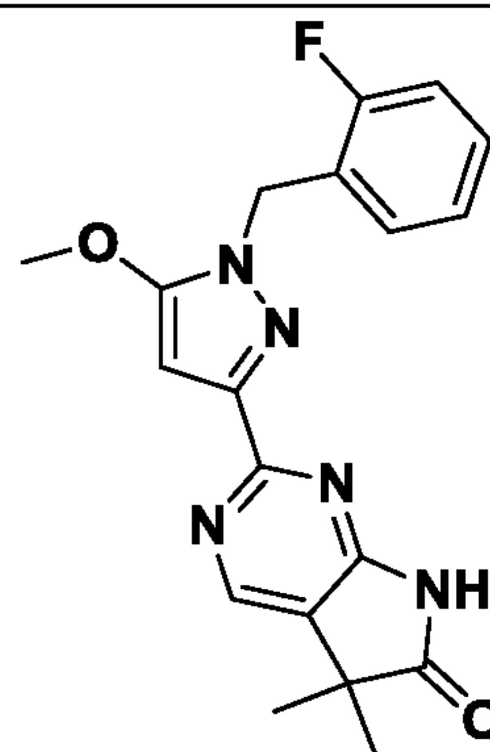
I-22
