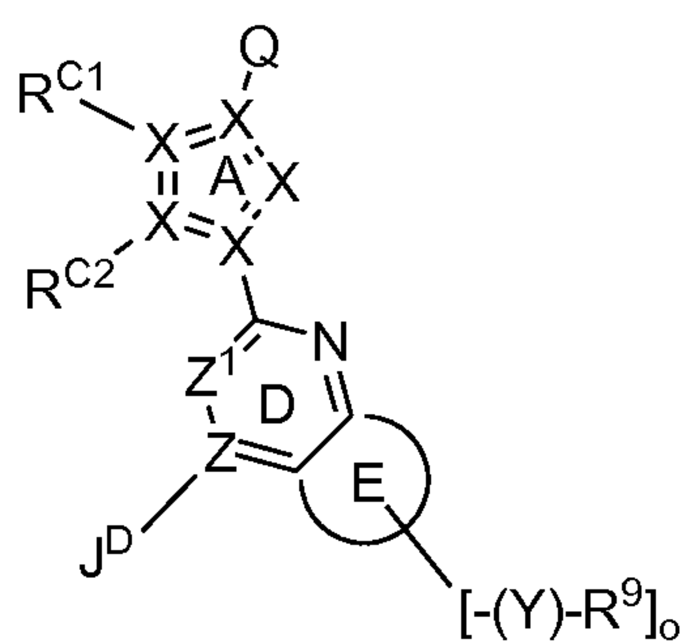
Formula I-a
