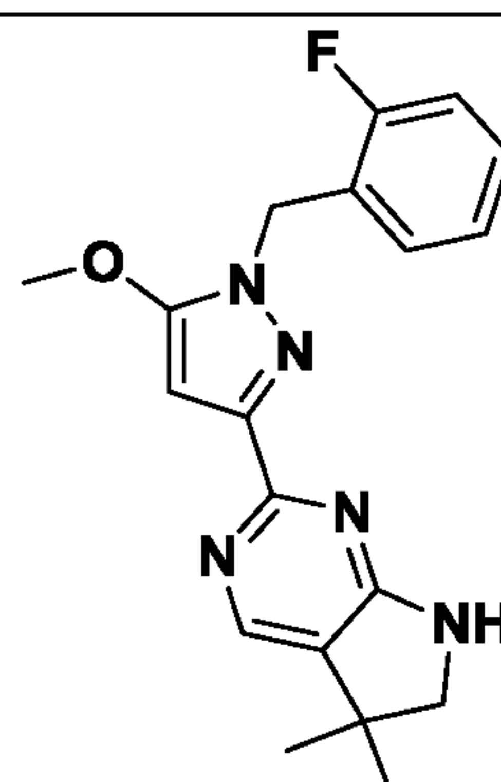
I-27
