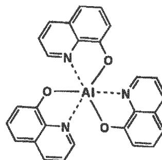
Alq 3
