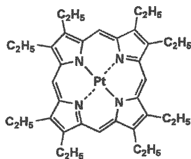
Pt-3
