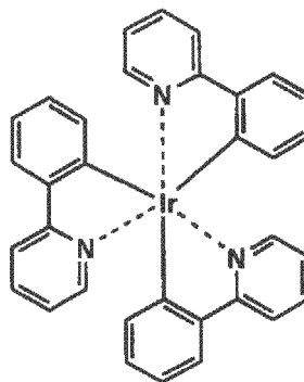
Ir(ppy) 3
