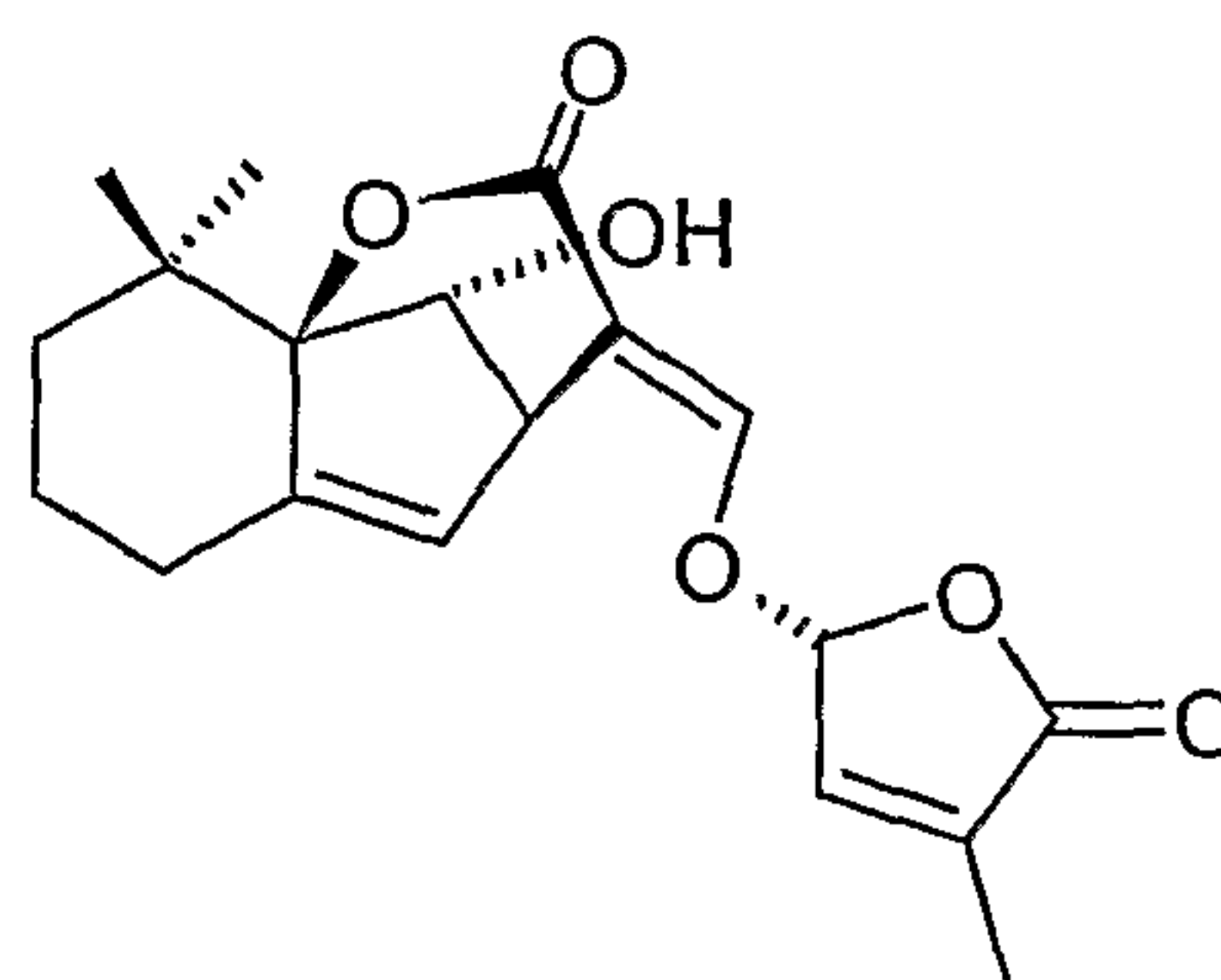
Sorgolactone (Hauck et al., J. Plant Physiol., 1992, 139:474)
