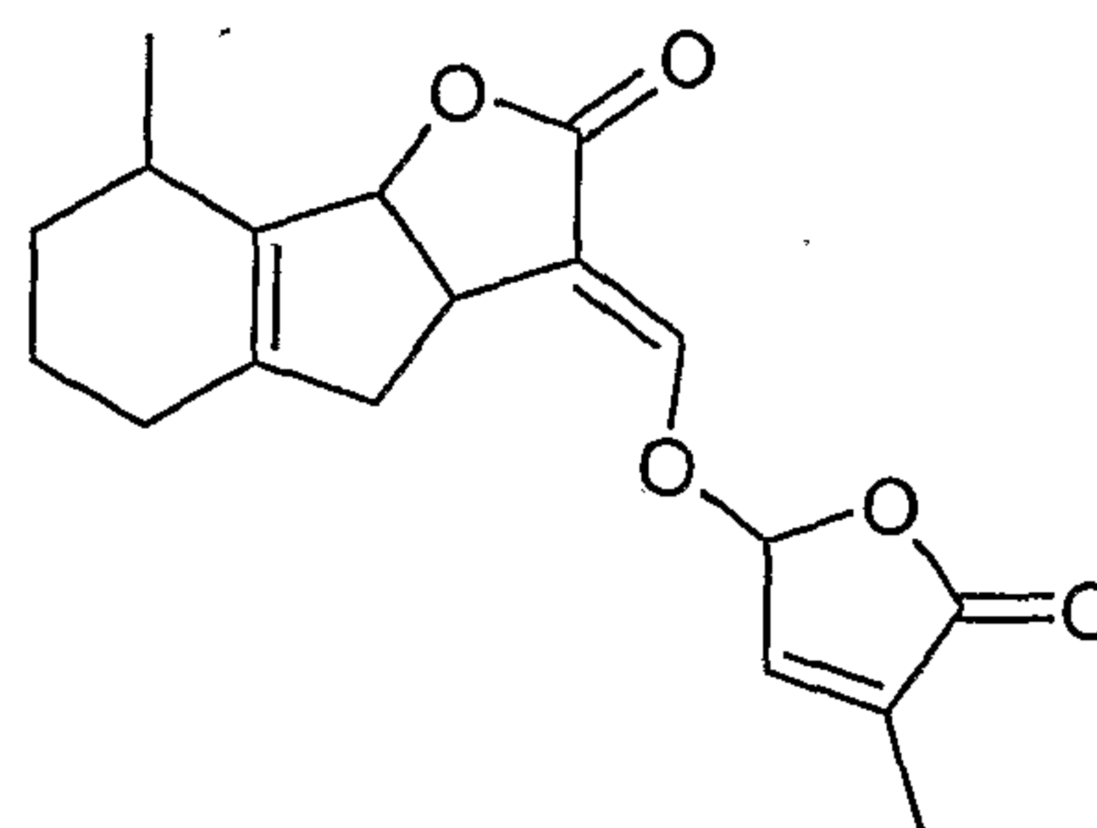
Sorgolactone (Hauck et al., J. Plant Physiol., 1992, 139:474)
