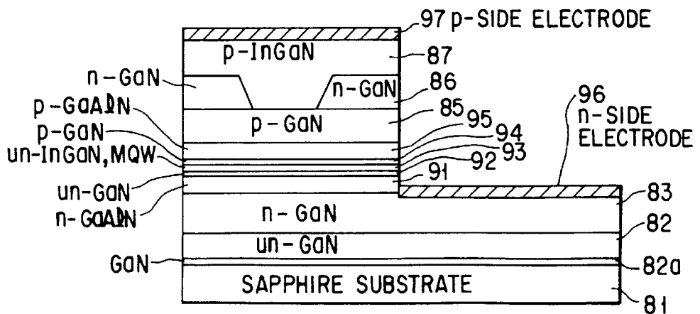
FIG. 30C
