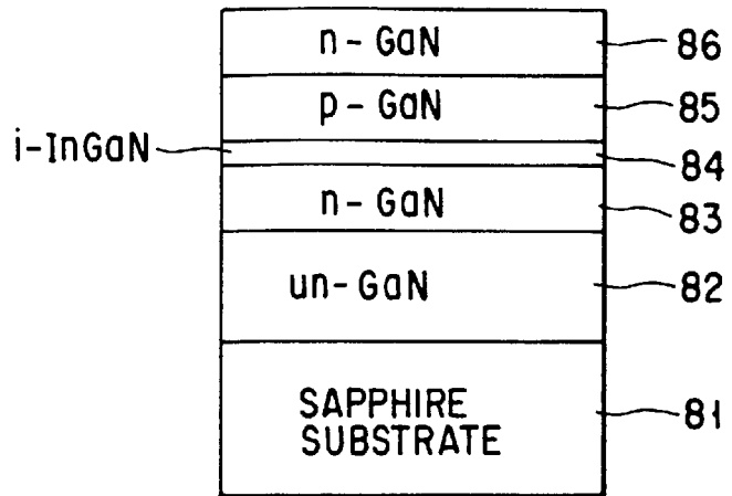
FIG. 26A
