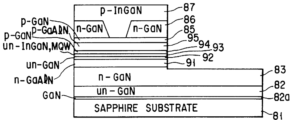
FIG. 30B
