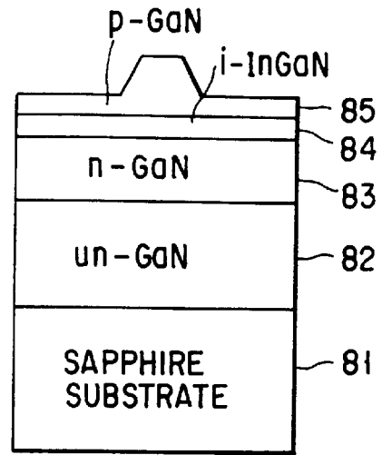
FIG. 34B
