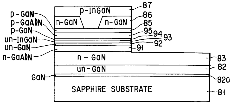
FIG. 30A
