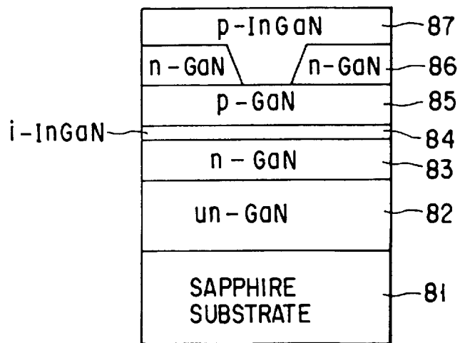
FIG. 26C
