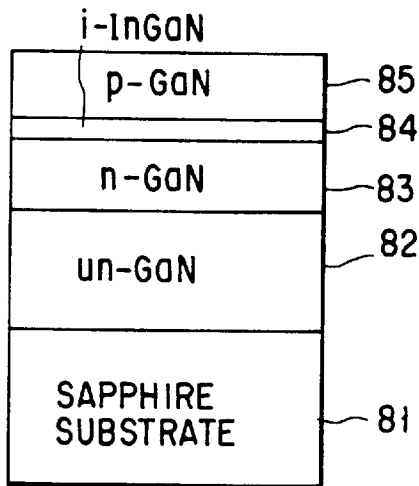
FIG. 34A
