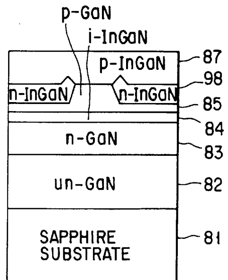
FIG. 34D
