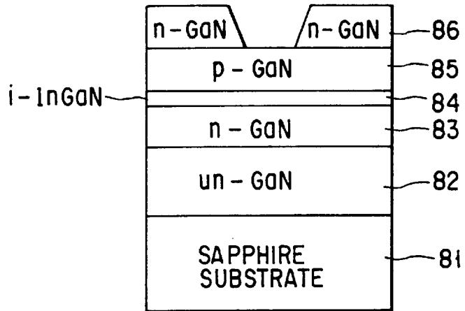
FIG. 26B
