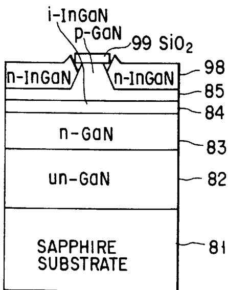
FIG. 34C
