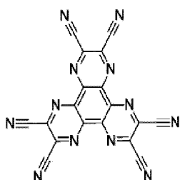
HIL : HAT-CN
