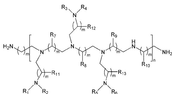
[Formule chimique 1]
