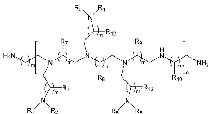
Chemische Formel 1
