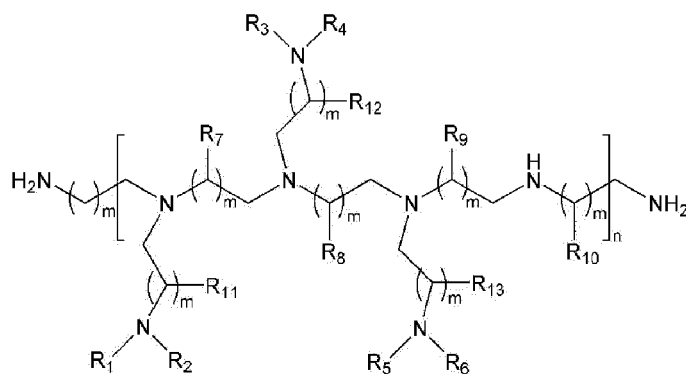
Chemische Formel 1
