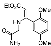
(Z)-Ethyl 3-((2-amino-2-oxoethyl)amino)-3-(2,5-dimethoxyphenyl)acrylate
