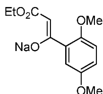
Sodium 1-(2,5-dimethoxyphenyl)-3-ethoxy-3-oxoprop-1-en-1-olate
