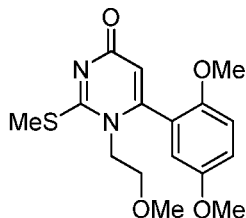
6-(2,5-dimethoxyphenyl)-1-(2-methoxyethyl)-2-(methylthio)pyrimidin-4(1H)-one
