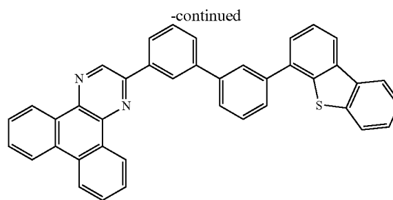
2mDBTPDBq-II
