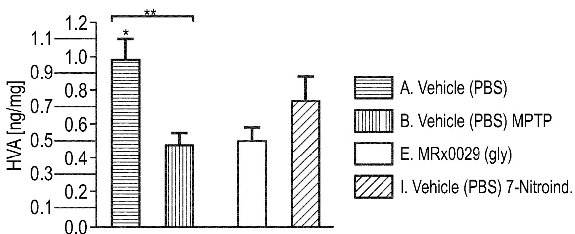
FIG. 12C HVA
