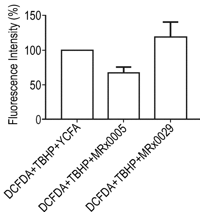
FIG. 14A Total ROS production
