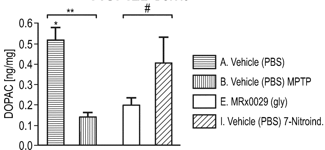
FIG. 12B DOPAC
