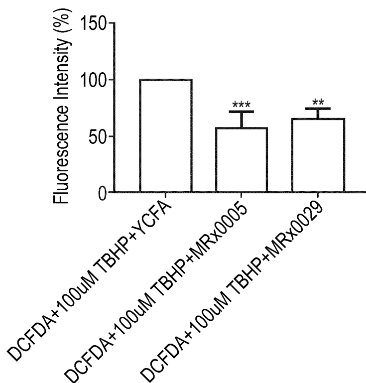
FIG. 14B Total ROS production
