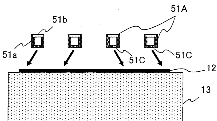
FIG.17B
