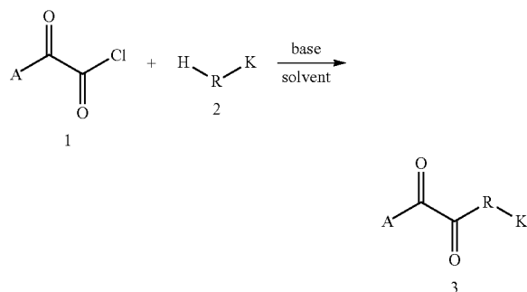
Scheme 1a
