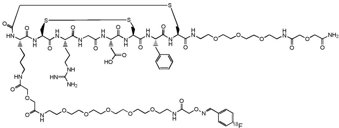
^{18}F -fluciclatide
