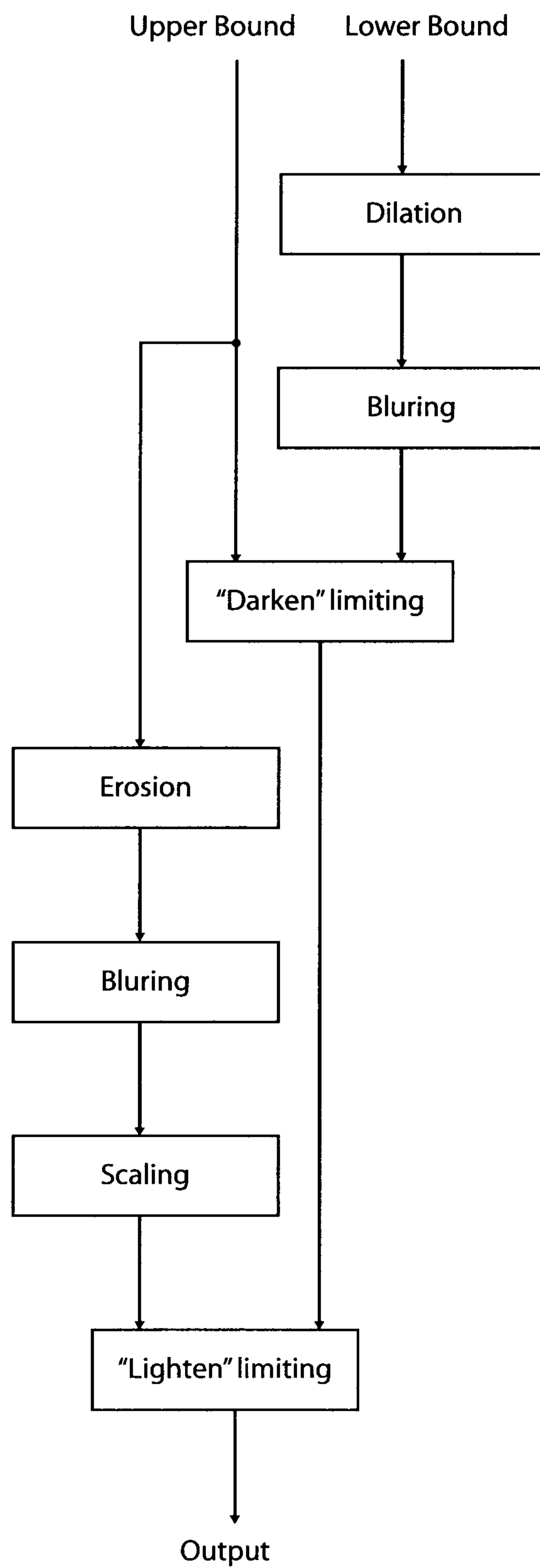
FIG. 20
