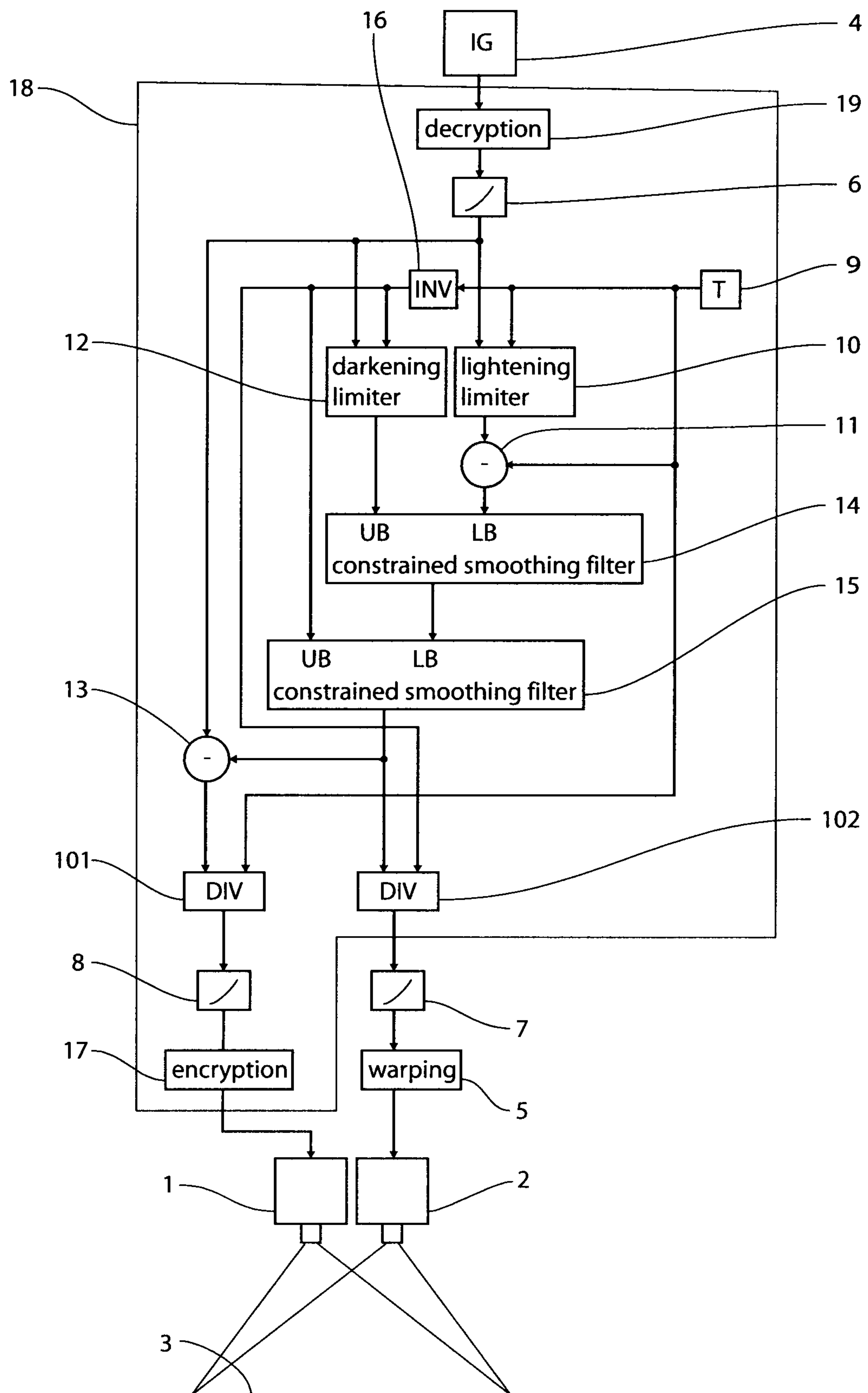
FIG. 12
