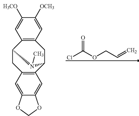
Scheme 26: (+)-Eschscholtzidine
