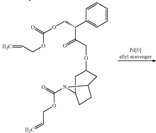
Scheme 26: (+)-Eschscholtzidine
