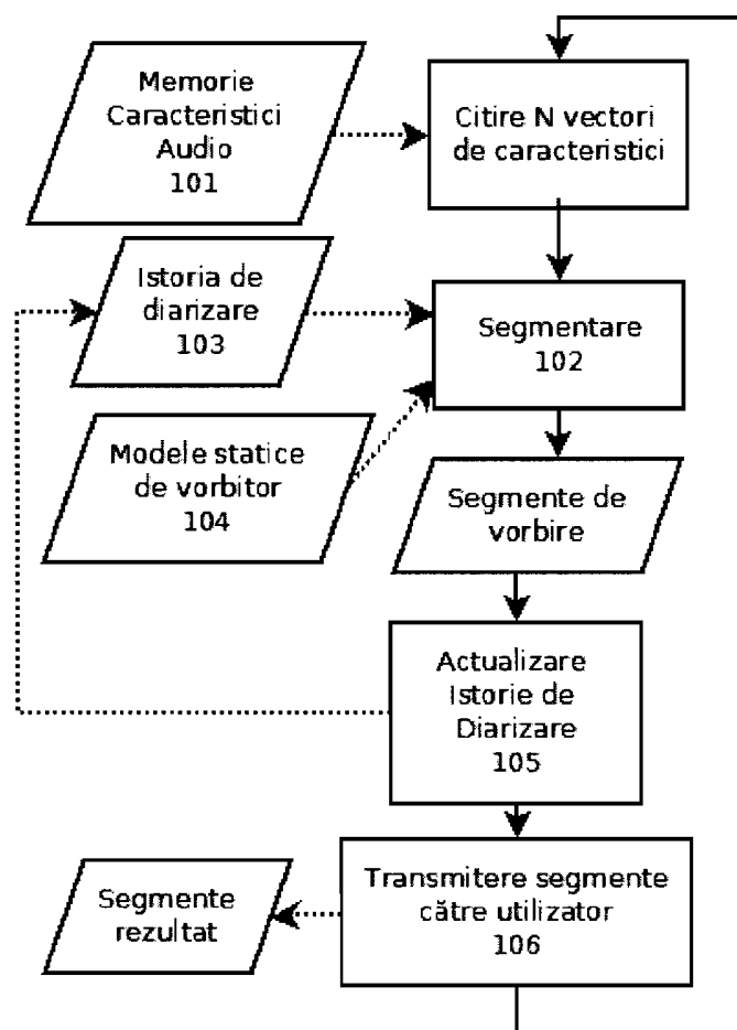
Figura 1: Metodă de diarizare
