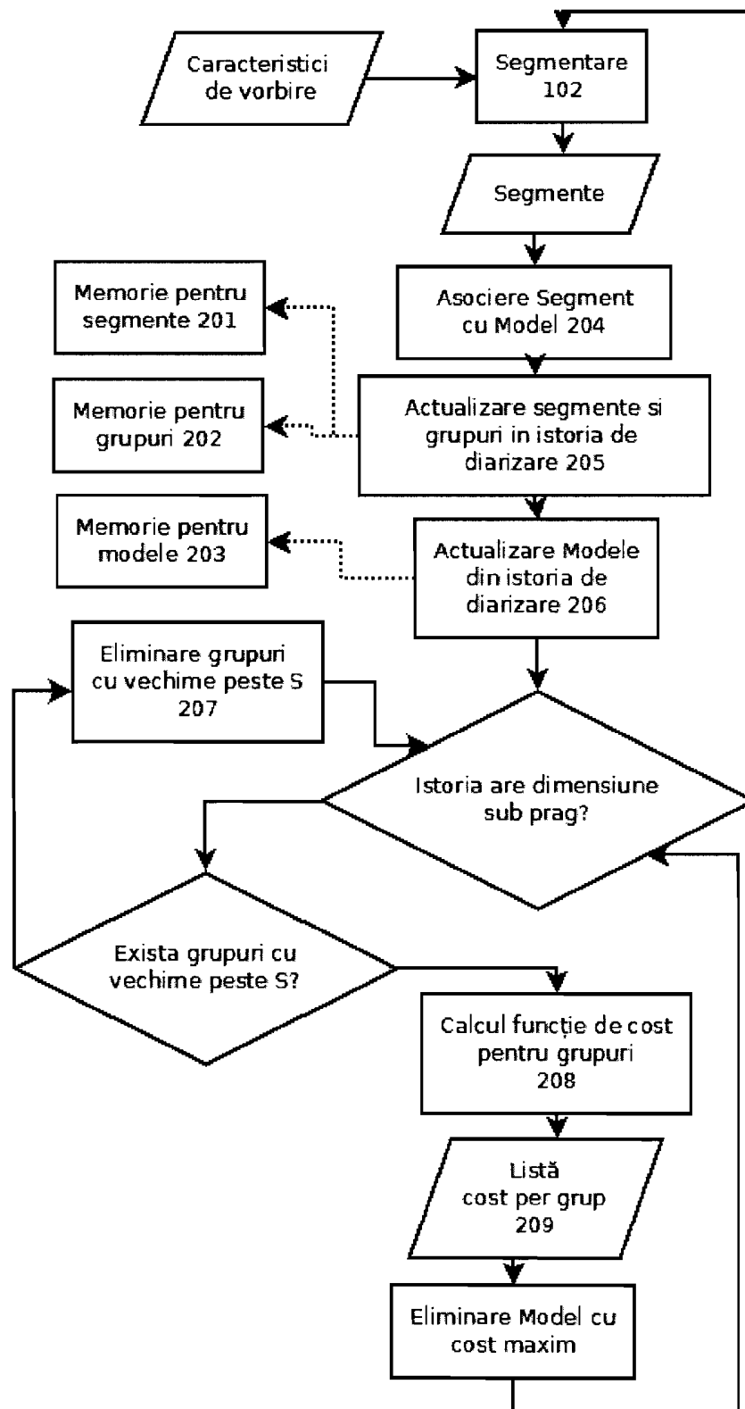
Figura 2: Gestiunea istoriei de diarizare
