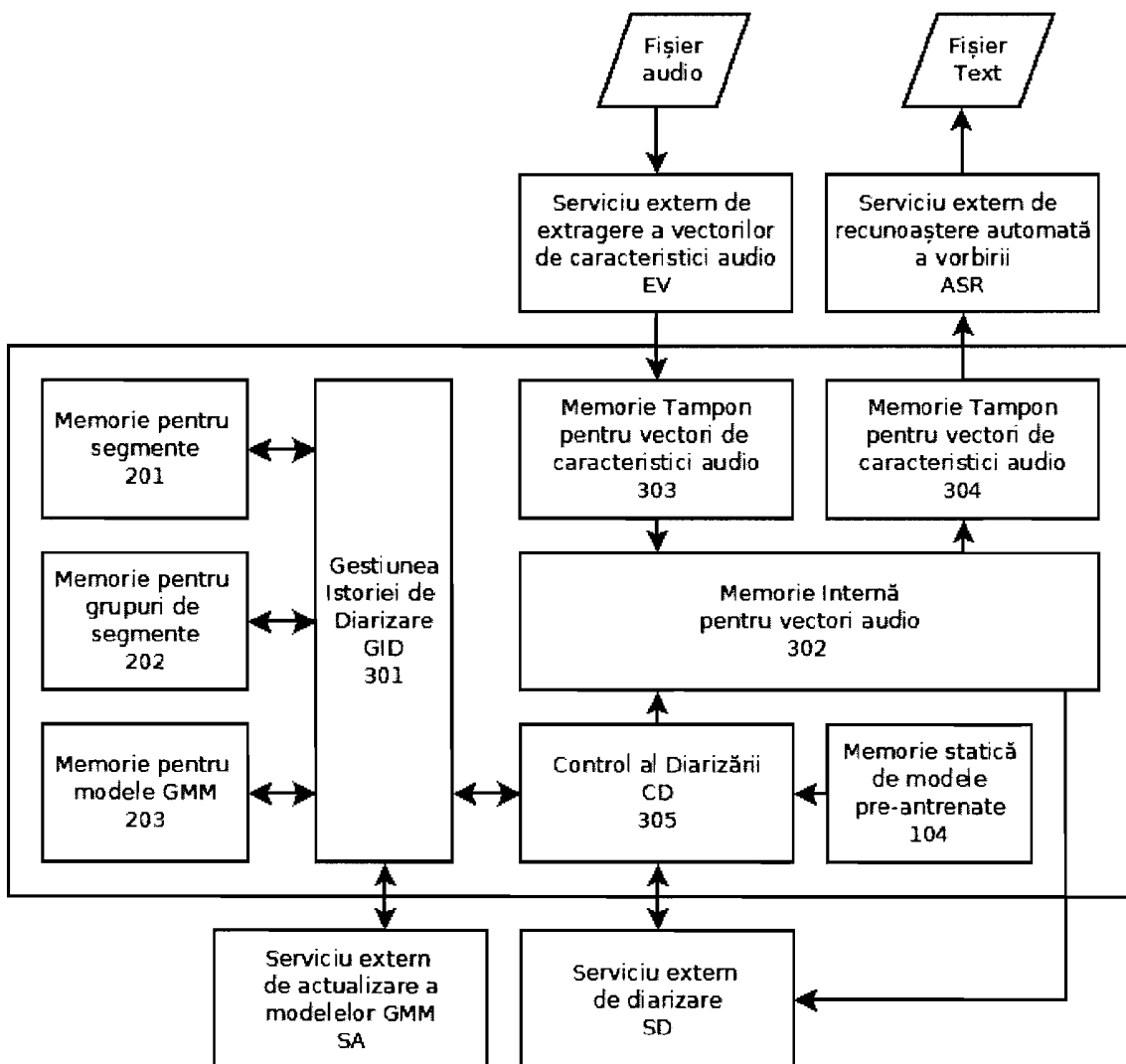
Figura 3: Sistem de diarizare în timp real
