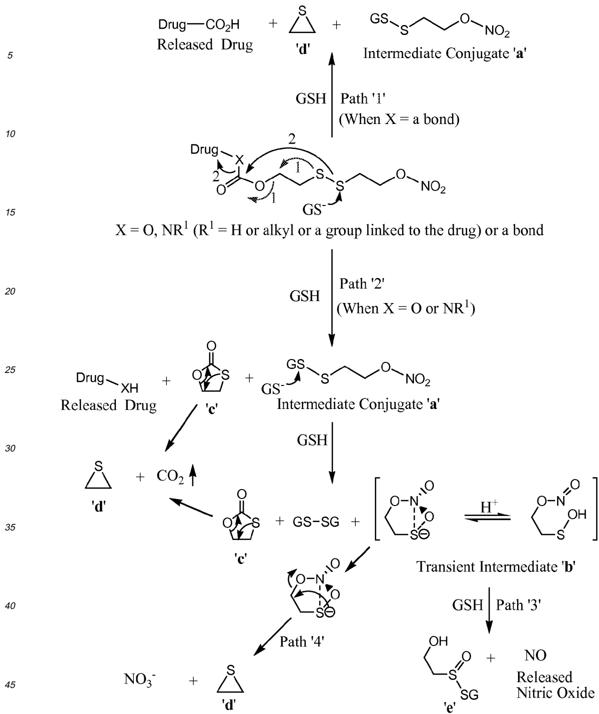
Scheme M1
