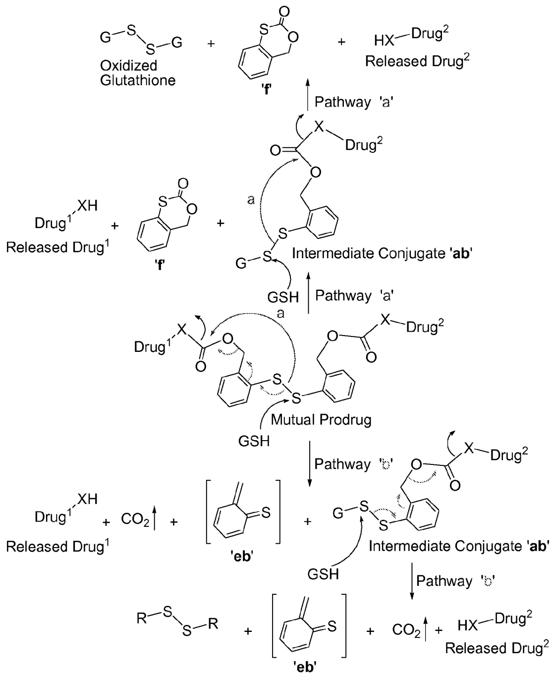
Scheme M6
