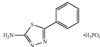
5-Phenyl-1,3,4-thiadiazol-2-amine Phosphate Salt
