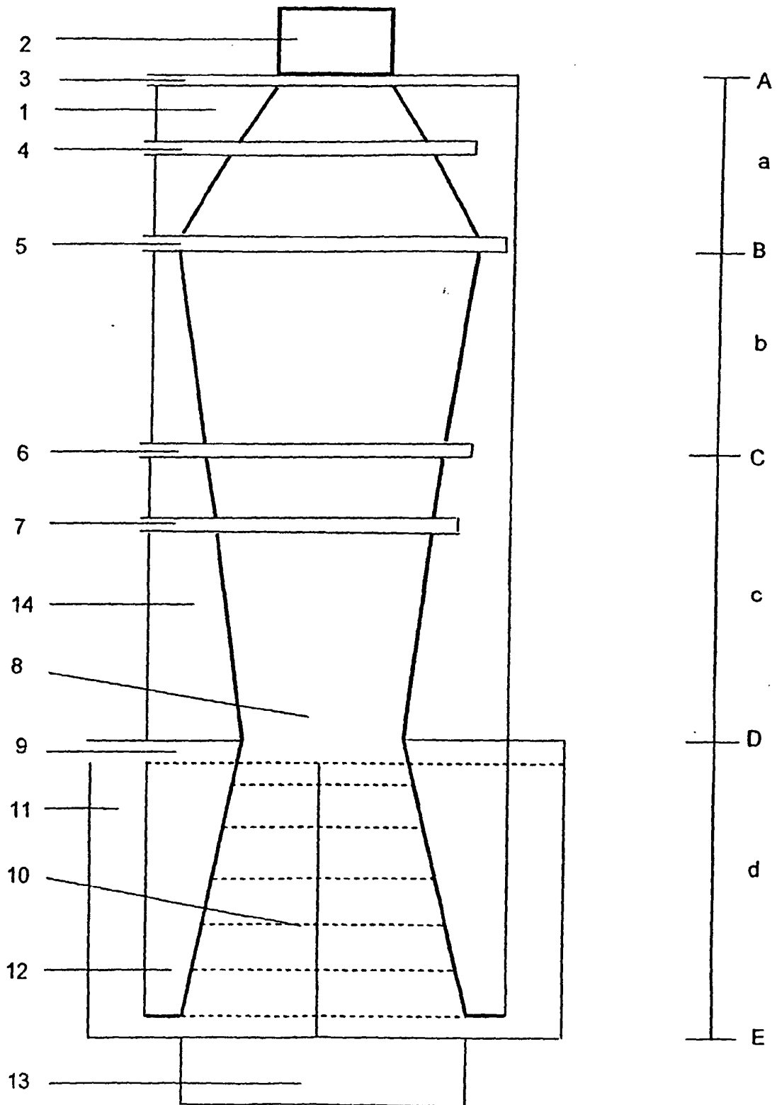
Figur 1 Längsschnitt durch den Reaktor
