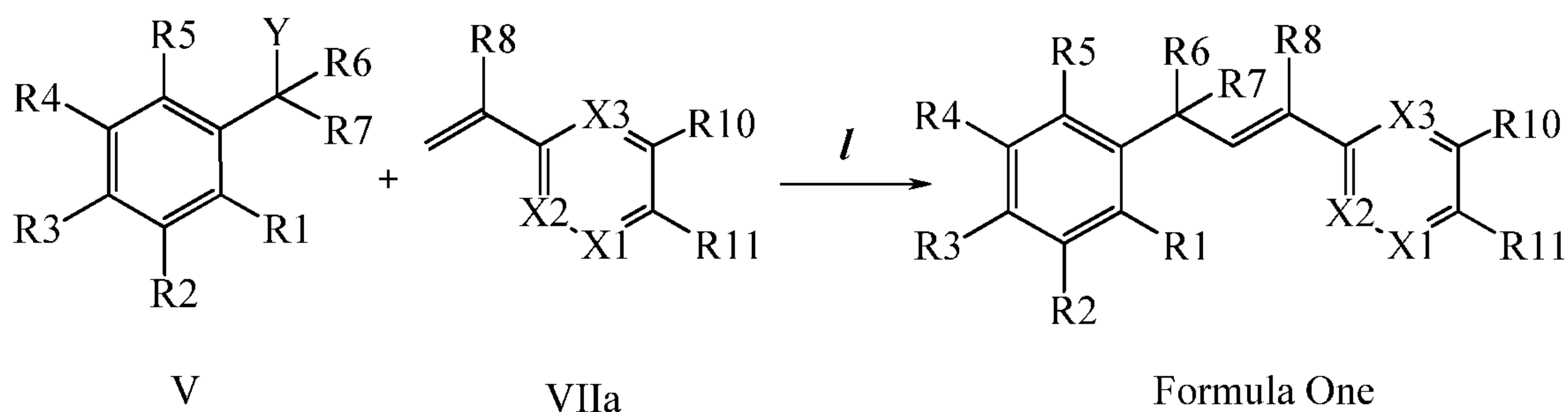
Scheme VI
