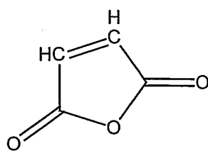
Maleic Anhydride
