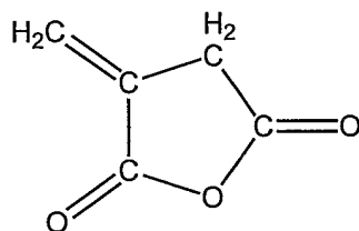
Itaconic Anhydride
