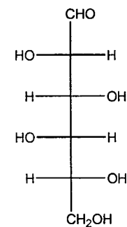
D-Idose
