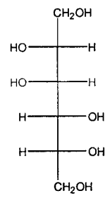
Mannitol
