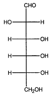
D-Altrose
