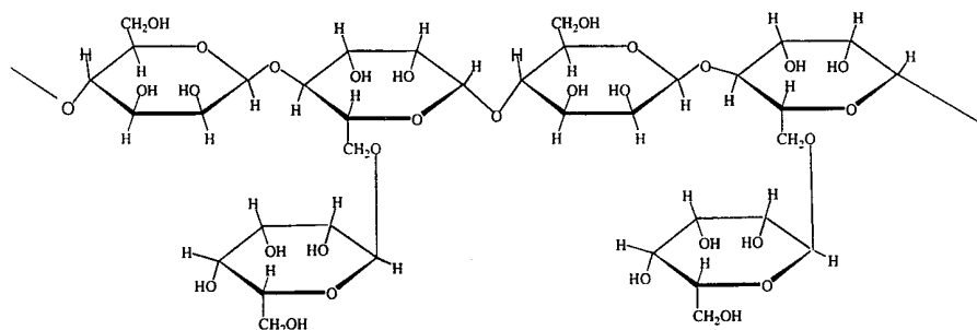
Guar Gum
