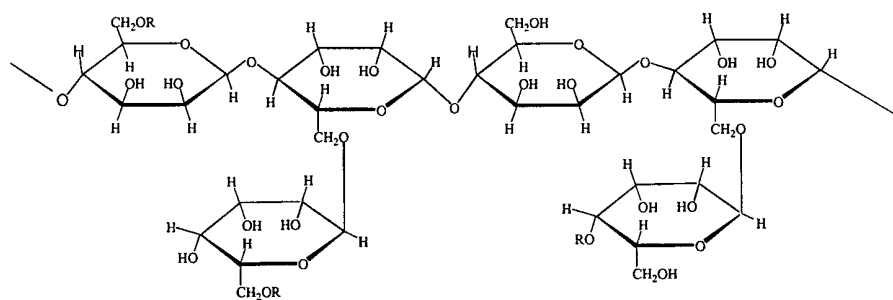
Guar Gum
