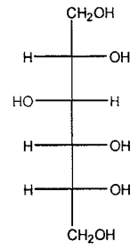
Sorbitol
