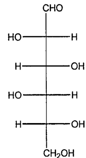
D-Talose
