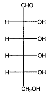
D-Allose
