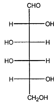
D-Galactose
