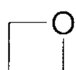
oxetane (oxetanyl)
