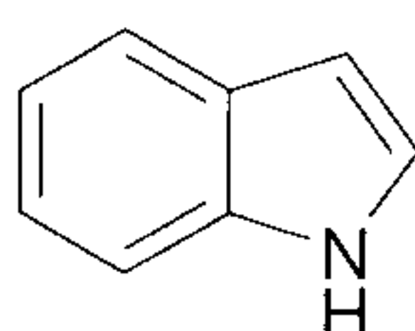
indole (indolyl)
