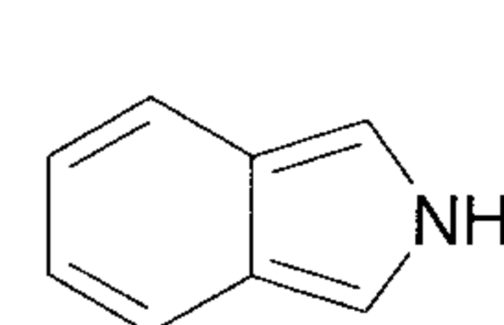
isoindole (isoindolyl)
