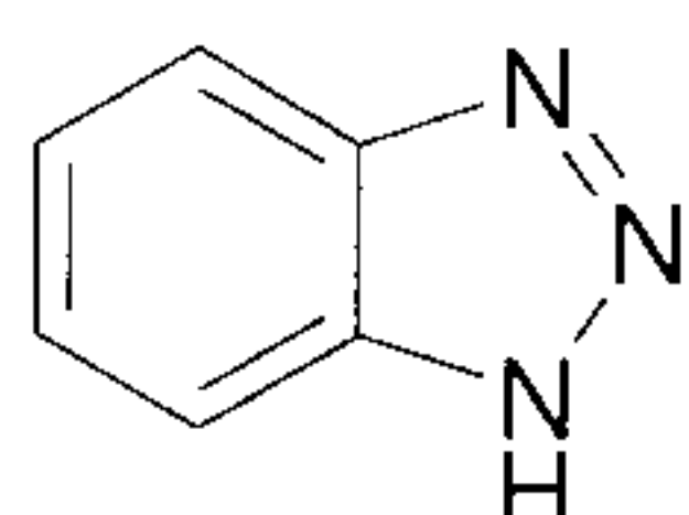
benzotriazole (benzotriazolyl)
