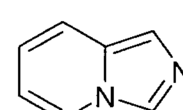
imidazo[1,5-a]pyridine (imidazo[1,5-a]pyridinyl)
