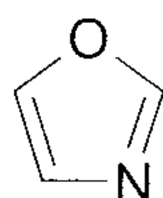
oxazole (oxazolyl)
