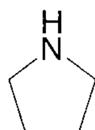
pyrrolidine (pyrrolidiny)
