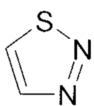
1-thia-2,3-diazole (1-thia-2,3-diazolyl)
