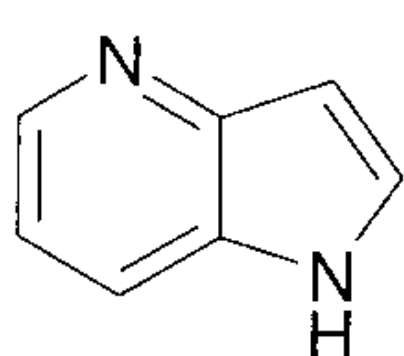
pyrrolo[3,2-b]pyridine (pyrrolo[3,2-b]pyridinyl)
