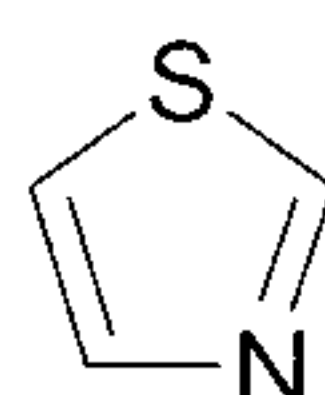
thiazolyl (thiazolyl)
