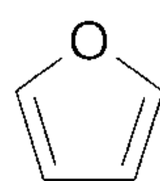
furan (furanyl)
