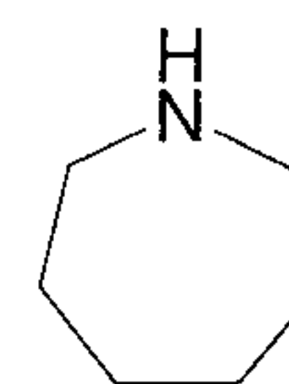
azepane (azepanyl)
