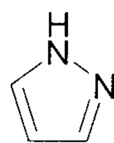
pyrazole (pyrazolyl)
