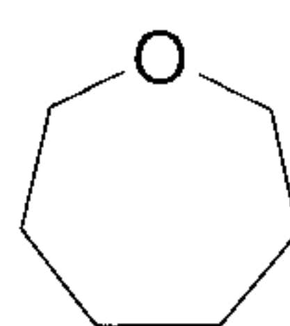
oxepane (oxepanyl)
