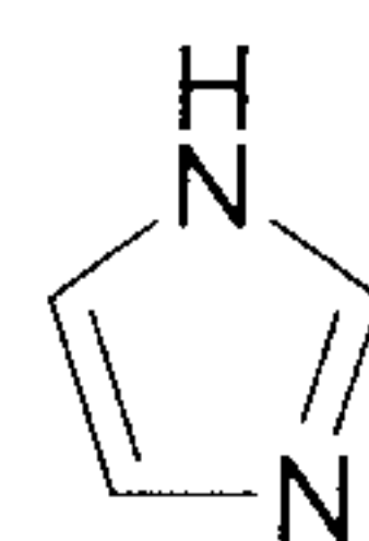
imidazole (imidazolyl)
