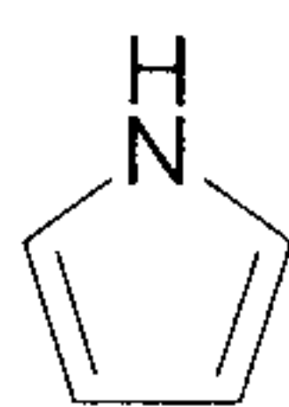
pyrrole (pyrrolyl)
