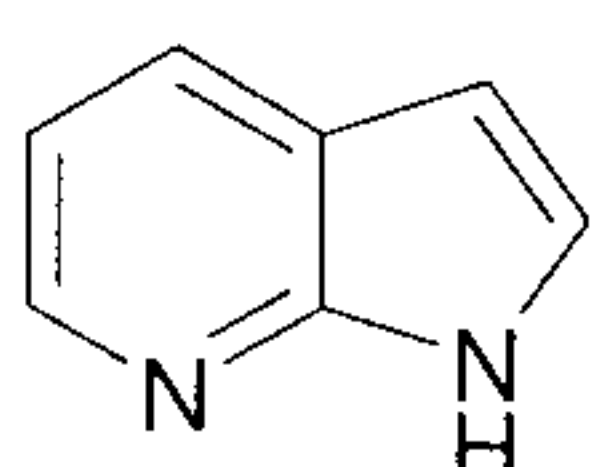
pyrrolo[2,3-b]pyridine (pyrrolo[2,3-b]pyridinyl)
