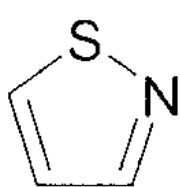
isothiazole (isothiazolyl)
