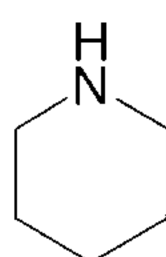
piperidine (piperidiny)
