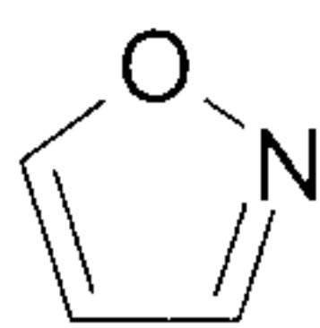
isoxazole (isoxazolyl)
