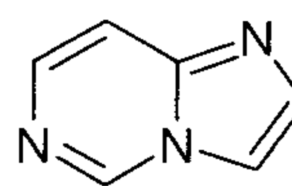
imidazo[1,2-c]pyrimidine (imidazo[1,2-c]pyrimidinyl)
