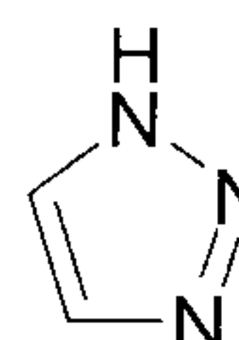
1,2,3-triazole (1,2,3-triazolyl)
