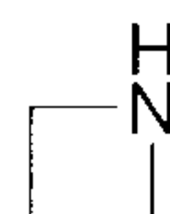
azetidine (azetidiny)
