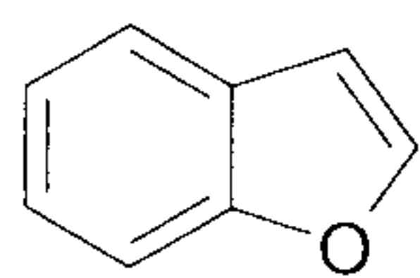
benzofuran (benzofuranyl)
