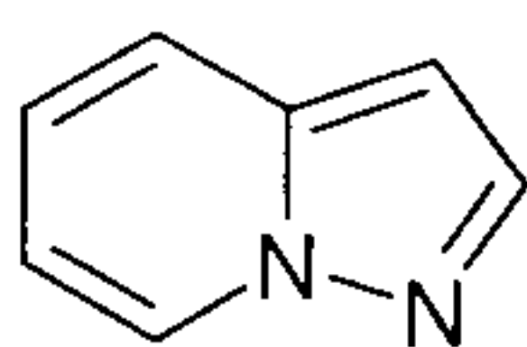
pyrazolo[1,5-a]pyridine (pyrazolo[1,5-a]pyridinyl)
