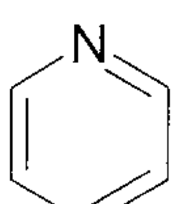
pyridine (pyridinyl)
