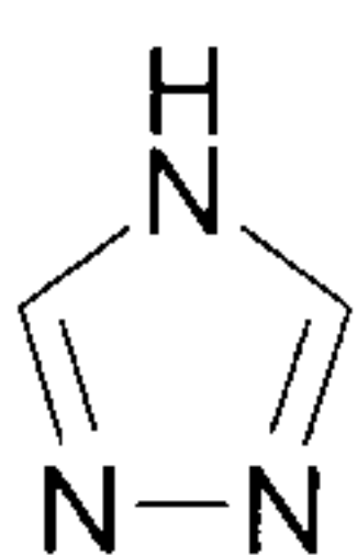
1,3,4-triazole (1,3,4-triazolyl)
