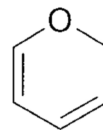
2H-pyran (2H-pyranyl)
