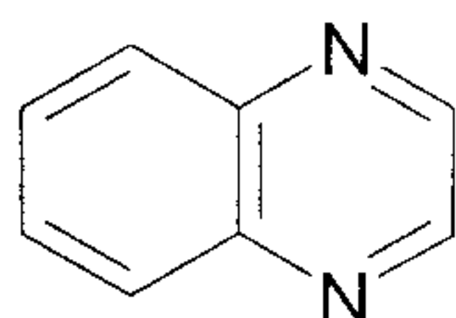
quinoxaline (quinoxalyl)
