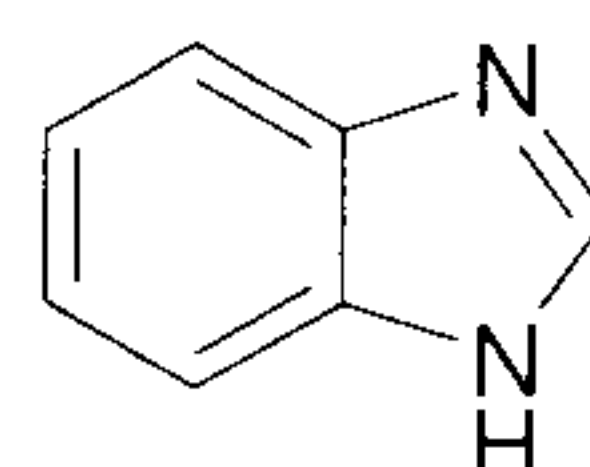
benzimidazole (benzimidazolyl)
