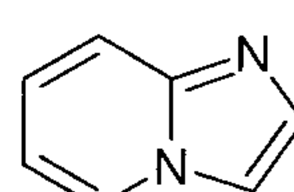
imidazo[1,2-a]pyridine (imidazo[1,2-a]pyridinyl)
