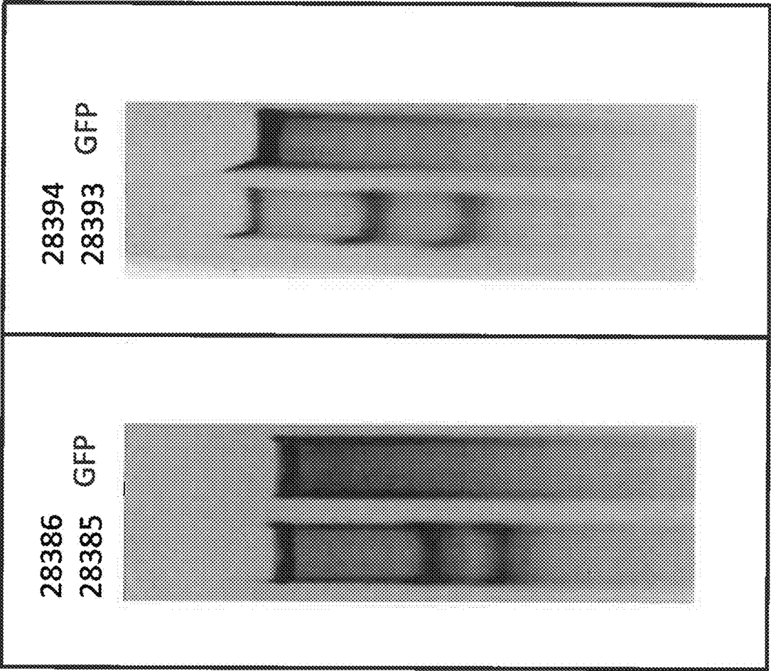
Figure 10B:TAP2
