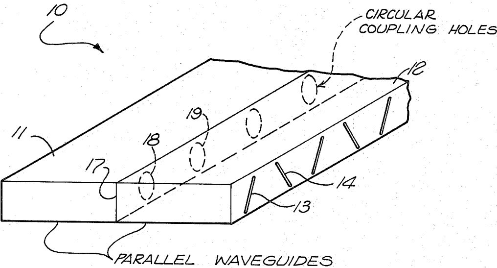
FIG. 1 MULTIBEAM SLOT ARRAY
