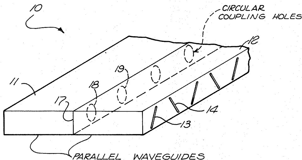
MULTIBEAM SLOT ARRAY
