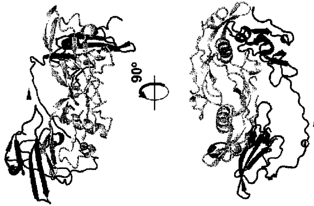
ActR-IIa/BMPR-Ia-v1 / BMP-2 complex
