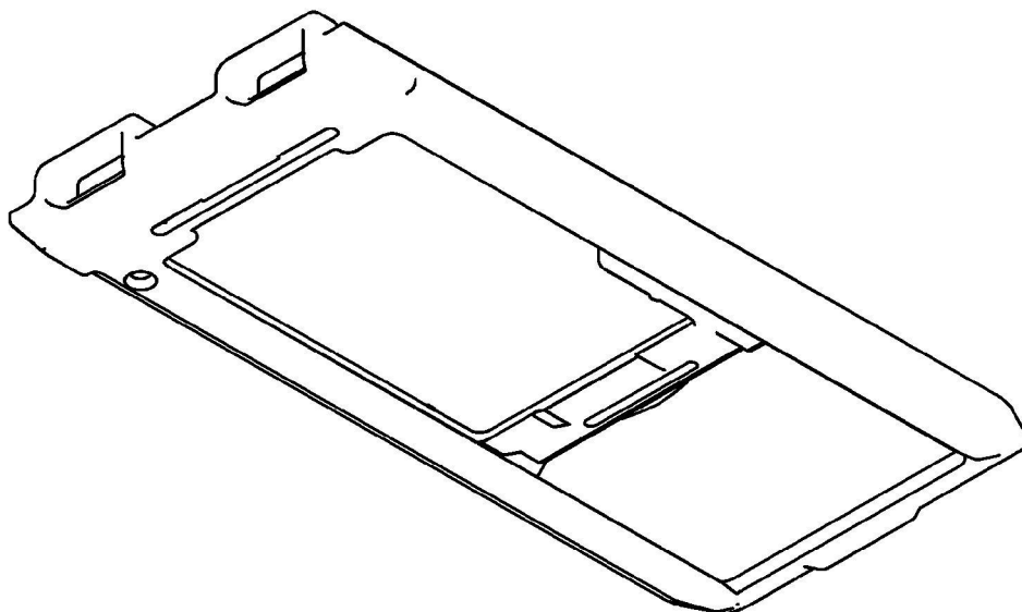
【立體圖 3】
