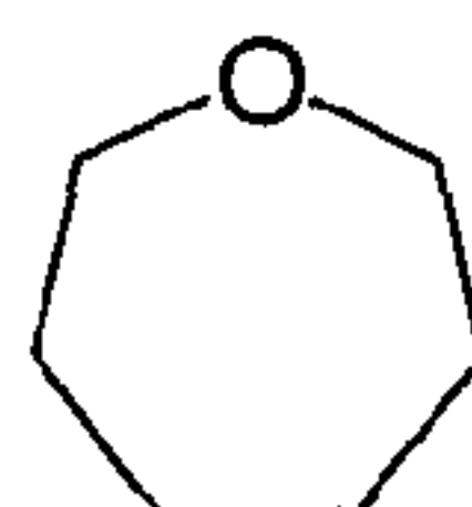
oxepane (oxepanyl)
