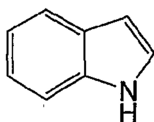
indole (indolyl)
