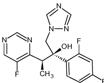
Voriconazole
