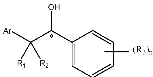
(II)
