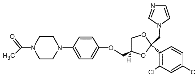
Ketoconazole
