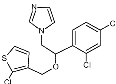
Tioconazole
