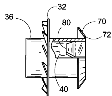
FIG. 5 SECTION A-A
