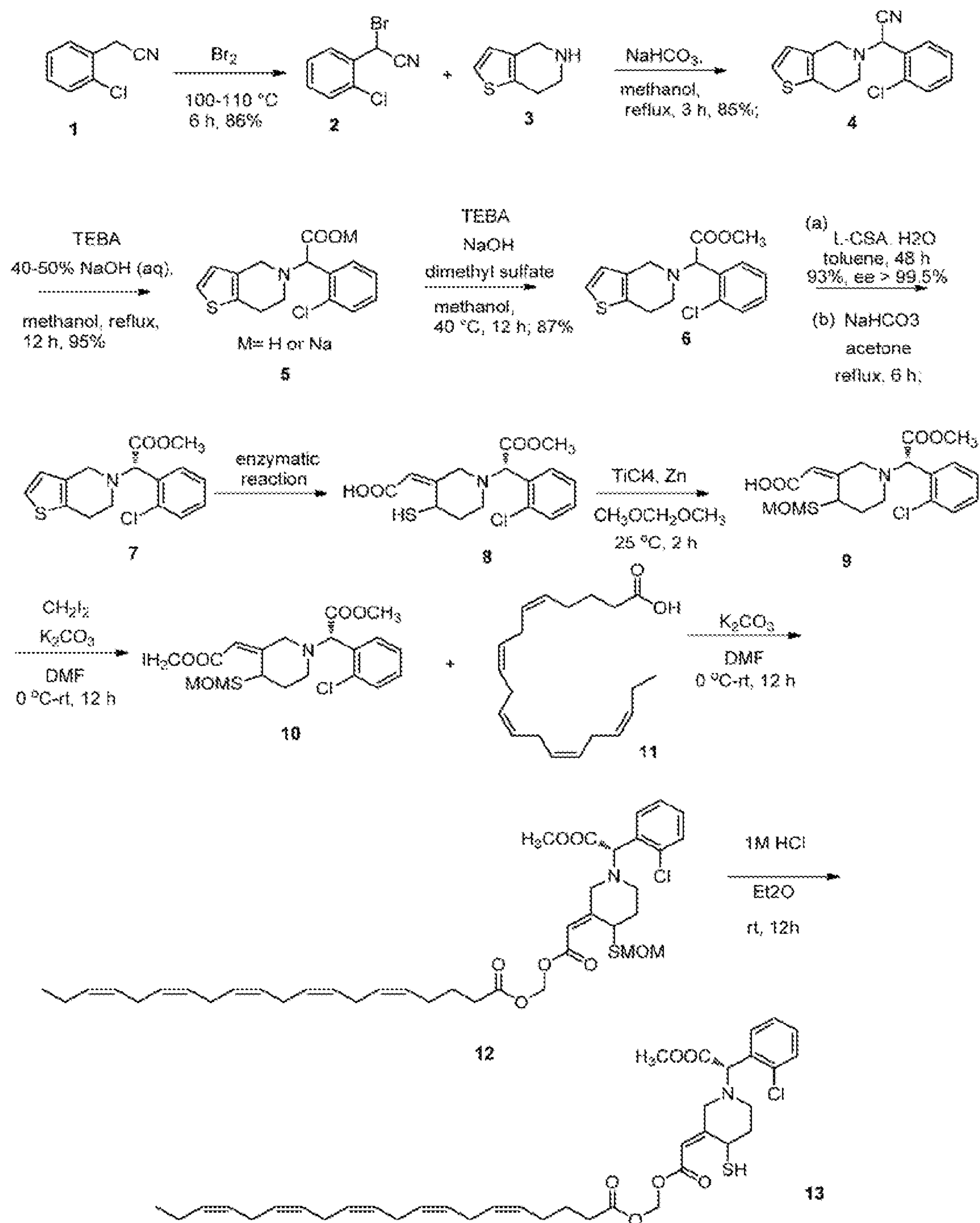
Scheme-1:
