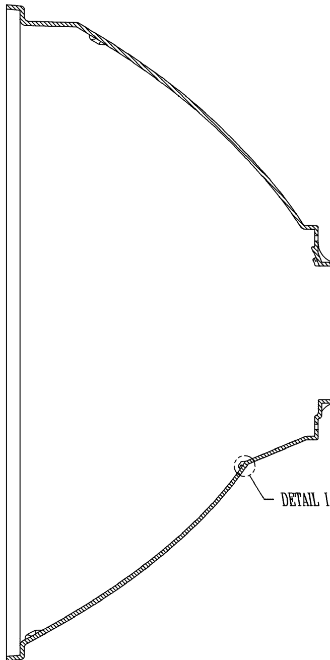
SECTION L-L Fig. 5P
