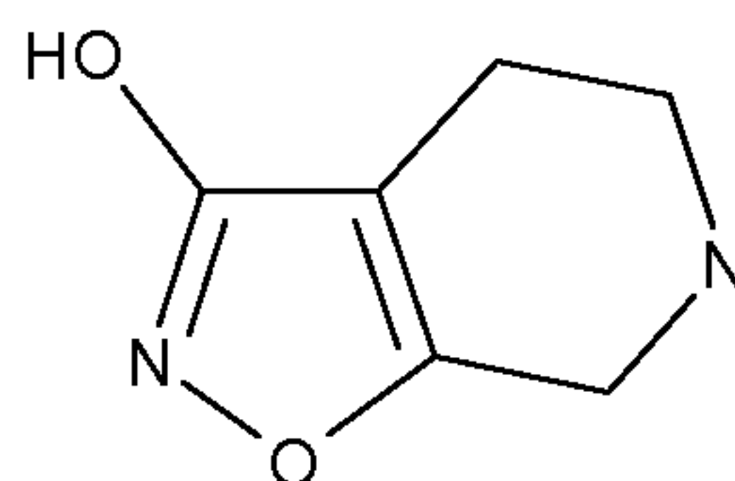
(gaboxadol)
