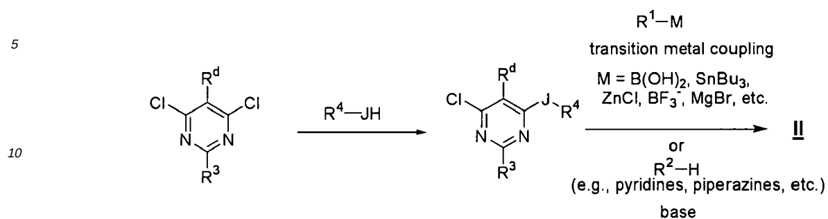
Scheme 2.b
