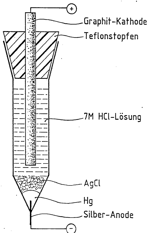
Galvanisches Silberhalogenid- Element
