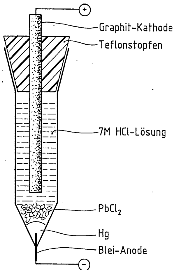
Galvanisches Bleihalogenid- Element
